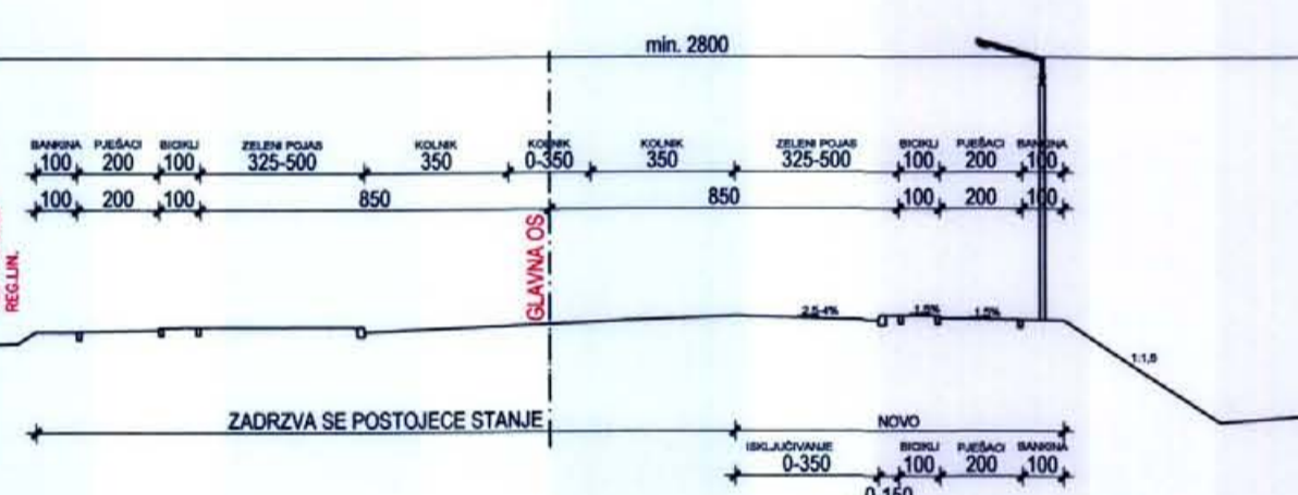
PRESJEK C-C, D 514 M 1:200
