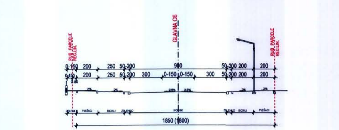
PRESJEK D-D, 2 4211 M 1:200
