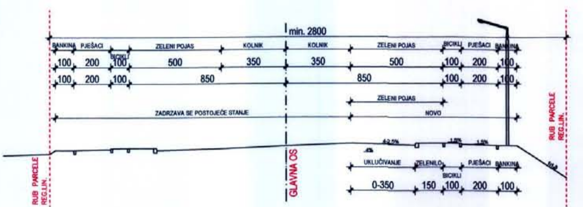
PRESJEK B-B, D 514 M 1:200
